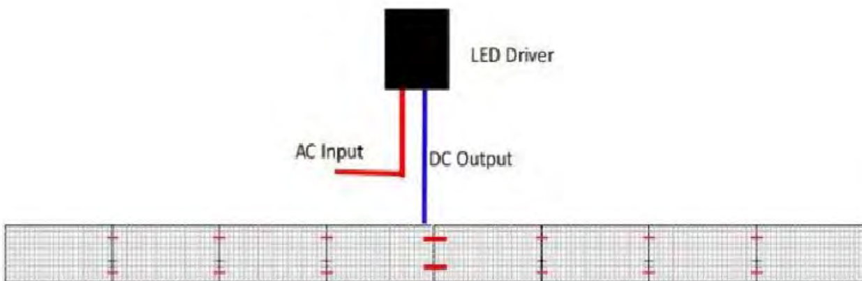
3. Connection method three/连接方式3
